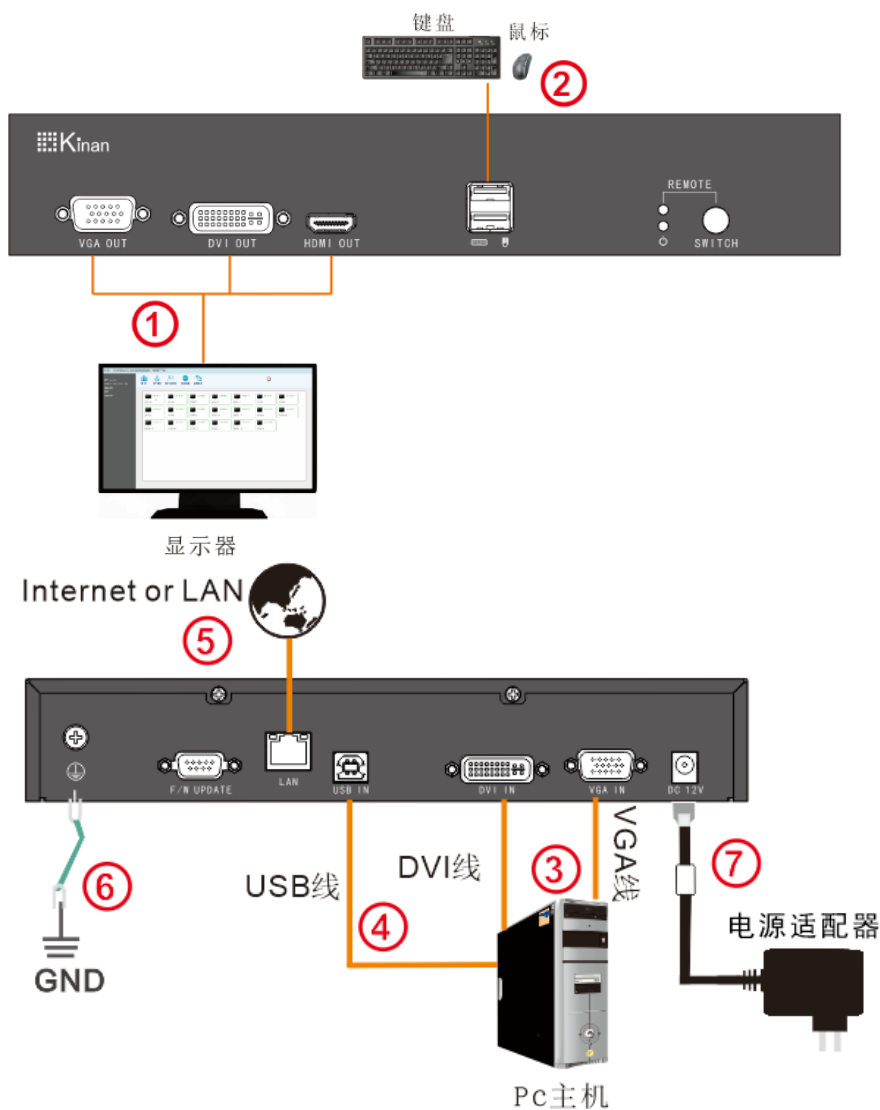
安装示意图
