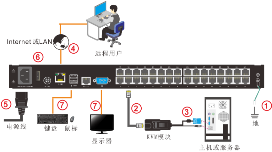
图 2-3 安装示意图
