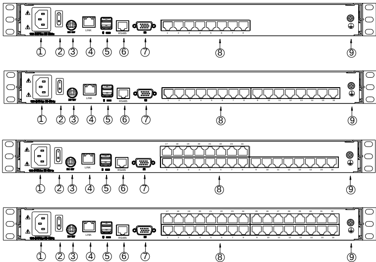
图 1-3 后视图
